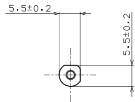
A - A (2 : 1)
