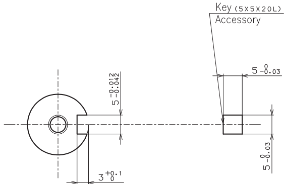
A - A (2 : 1)
